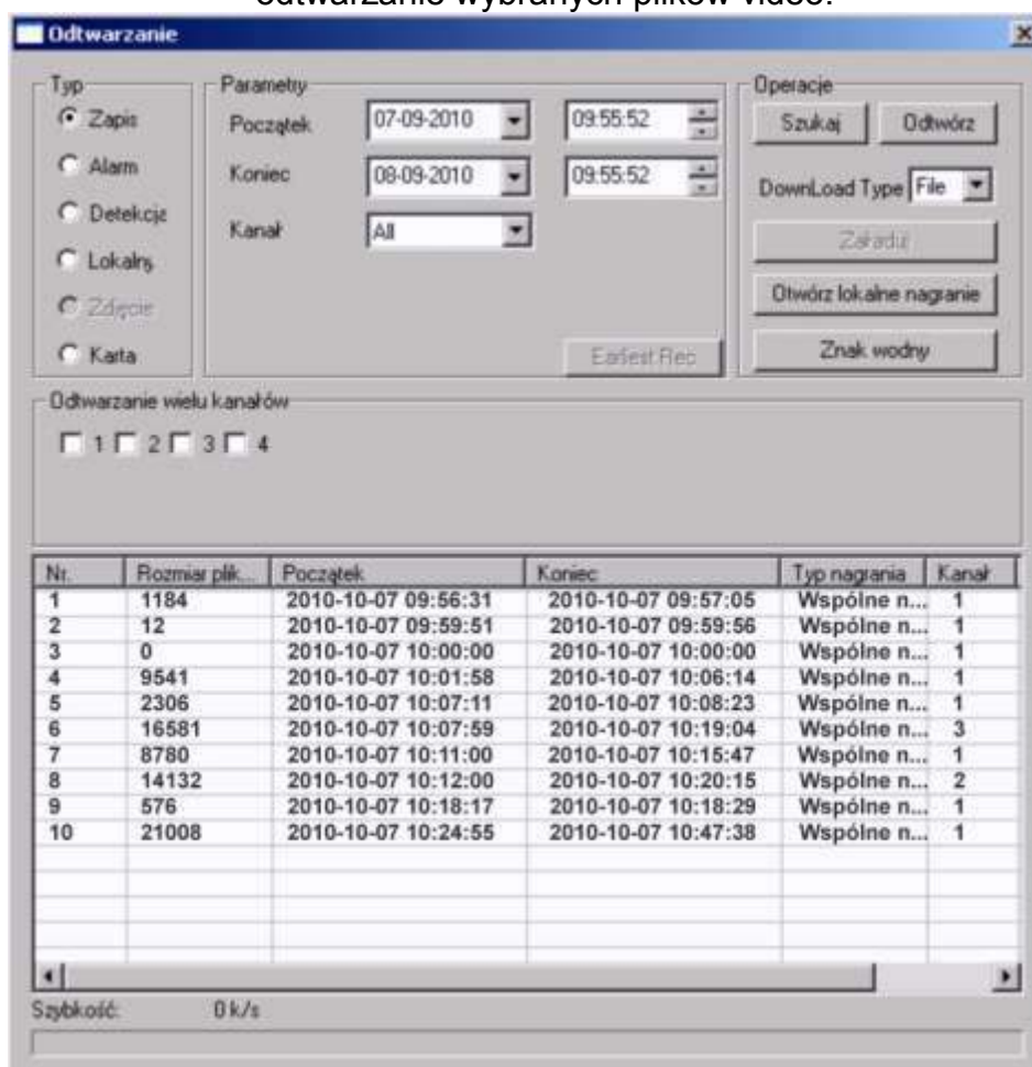
Rys. 7-58a. Interfejs Odtwarzanie.
