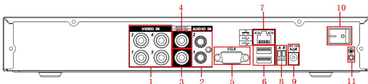
Rysunek 2-2a. Wygląd tylnego panelu rejestratora 4-kanalowego
