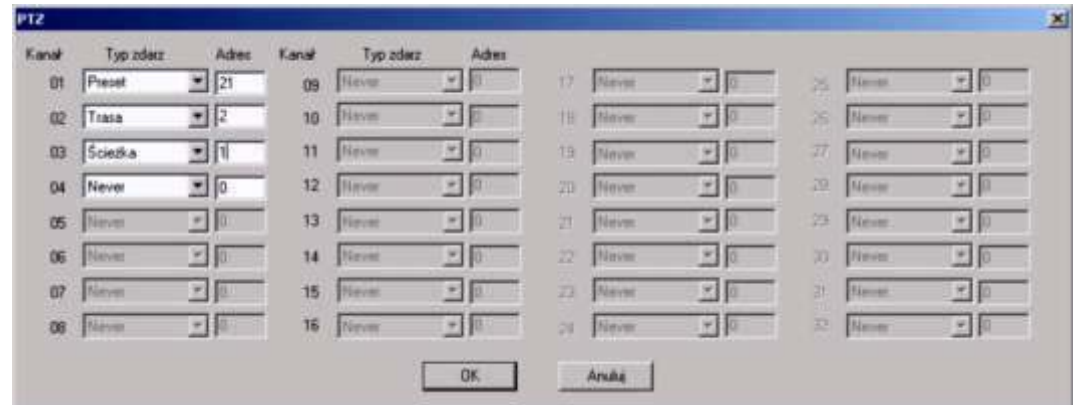
Rys. 7-38c. Ustawienia PTZ w reakcji na aktywację wejścia alarmowego.
