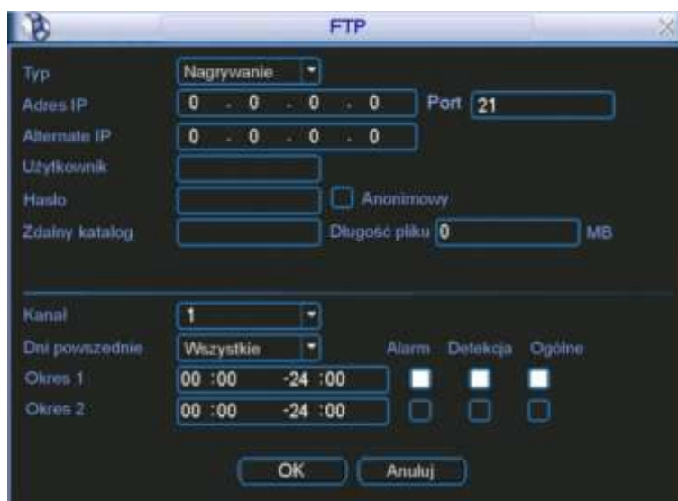
Rys. 5-16. Ustawianie FTP.
