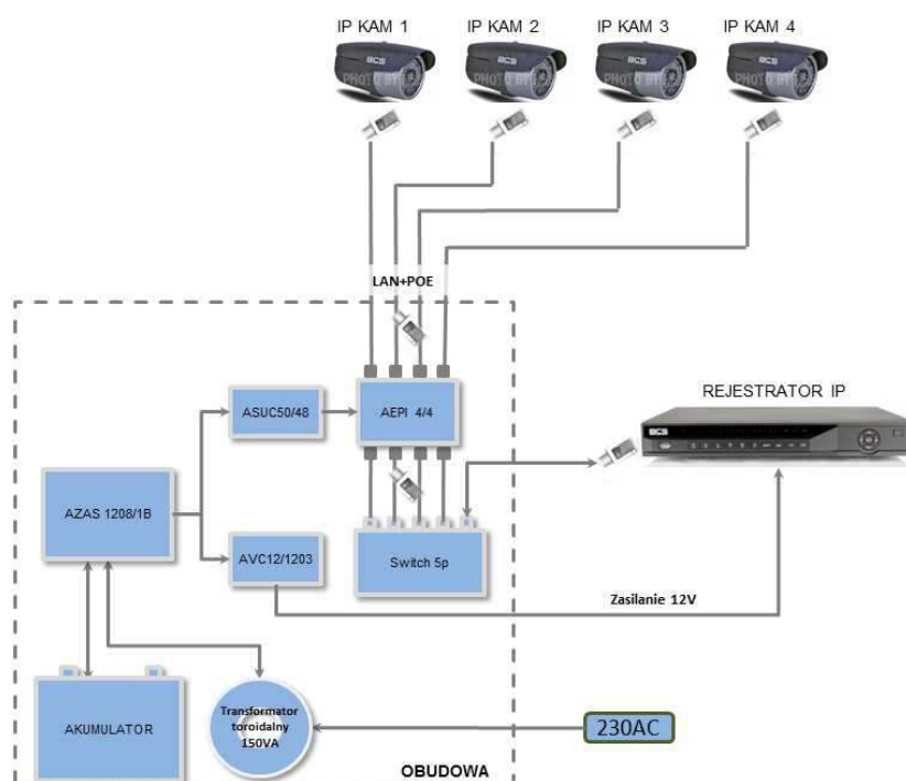
Schemat instalacji monitoringu dla 4 kamer IP BCS-UPS/IP4
