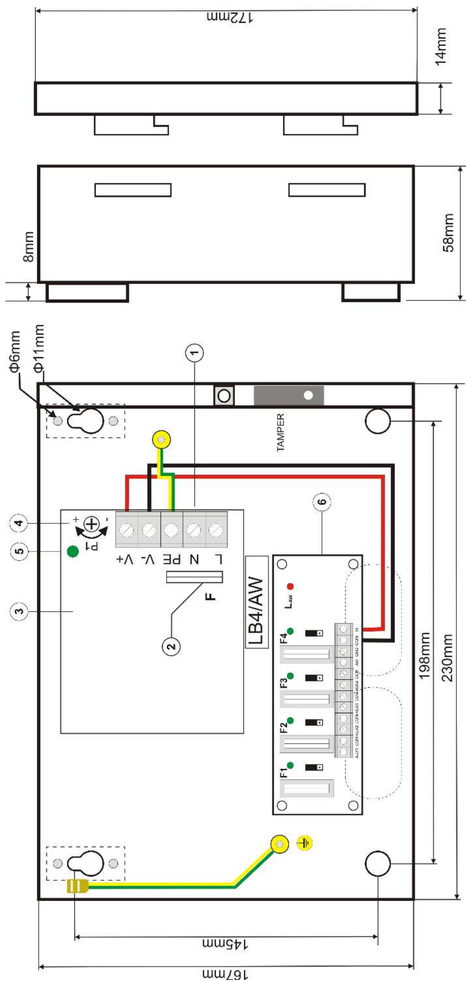
Rys.3. Widok zasilacza.
