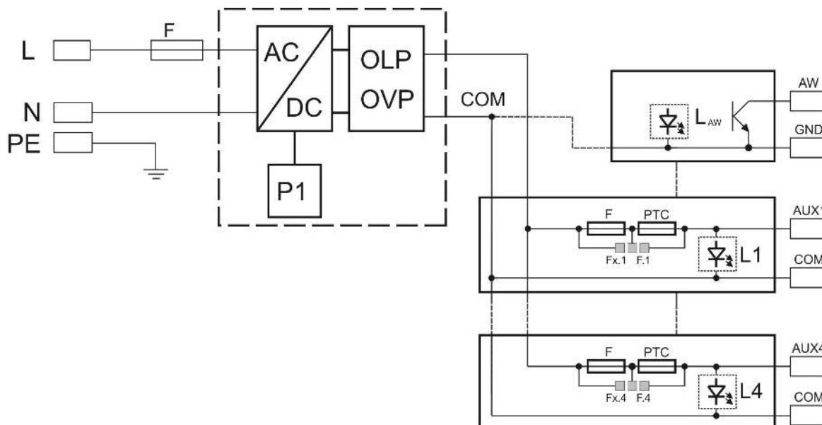
Rys.1. Schemat blokowy zasilacza.
