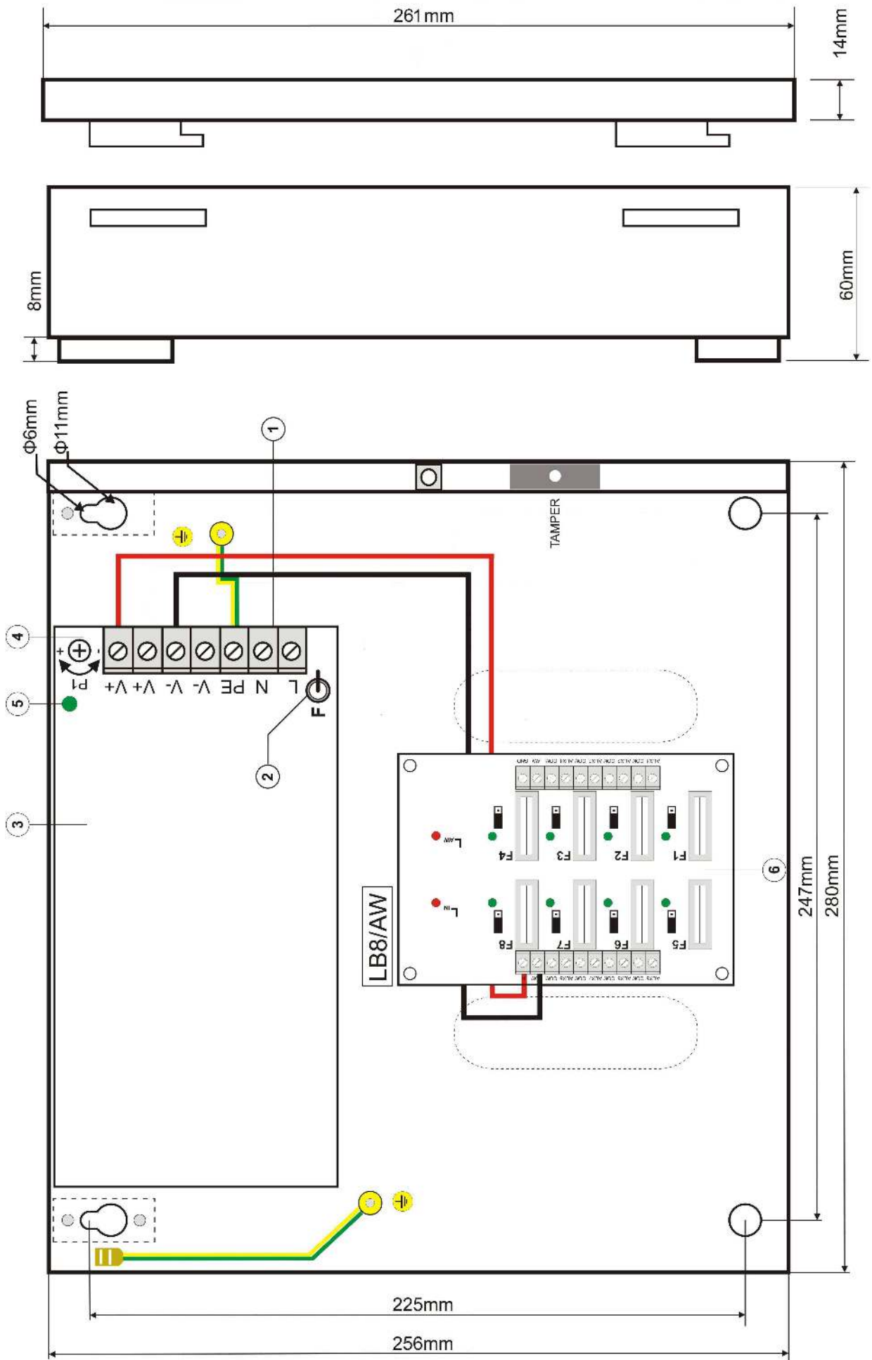
Rys.3. Widok zasilacza.
